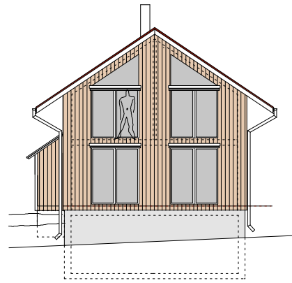
Ansicht Süd
