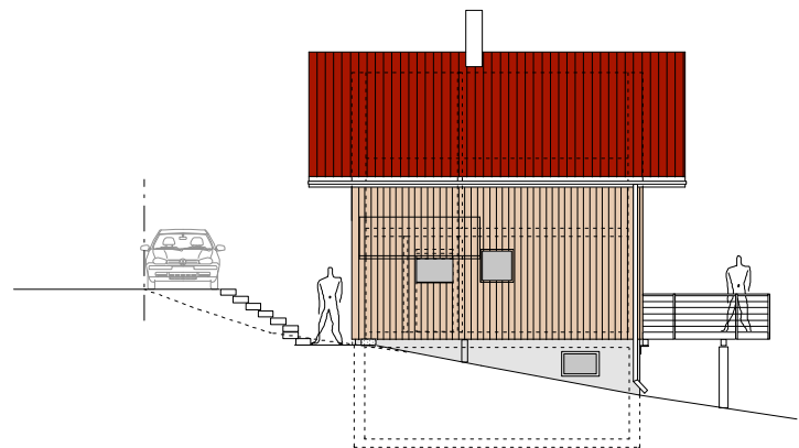
Ansicht West
