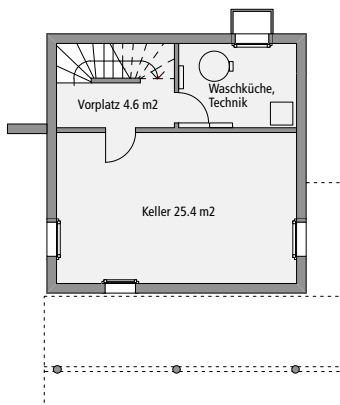
Untergeschoss
