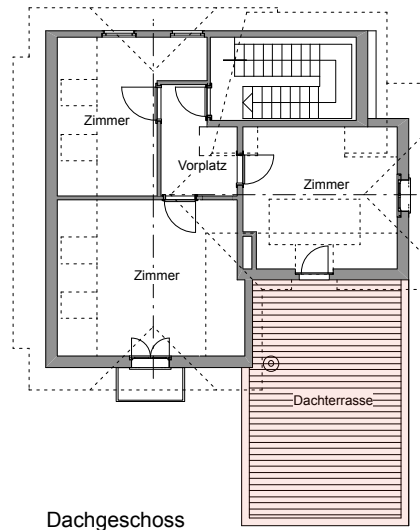
Dachgeschoss
